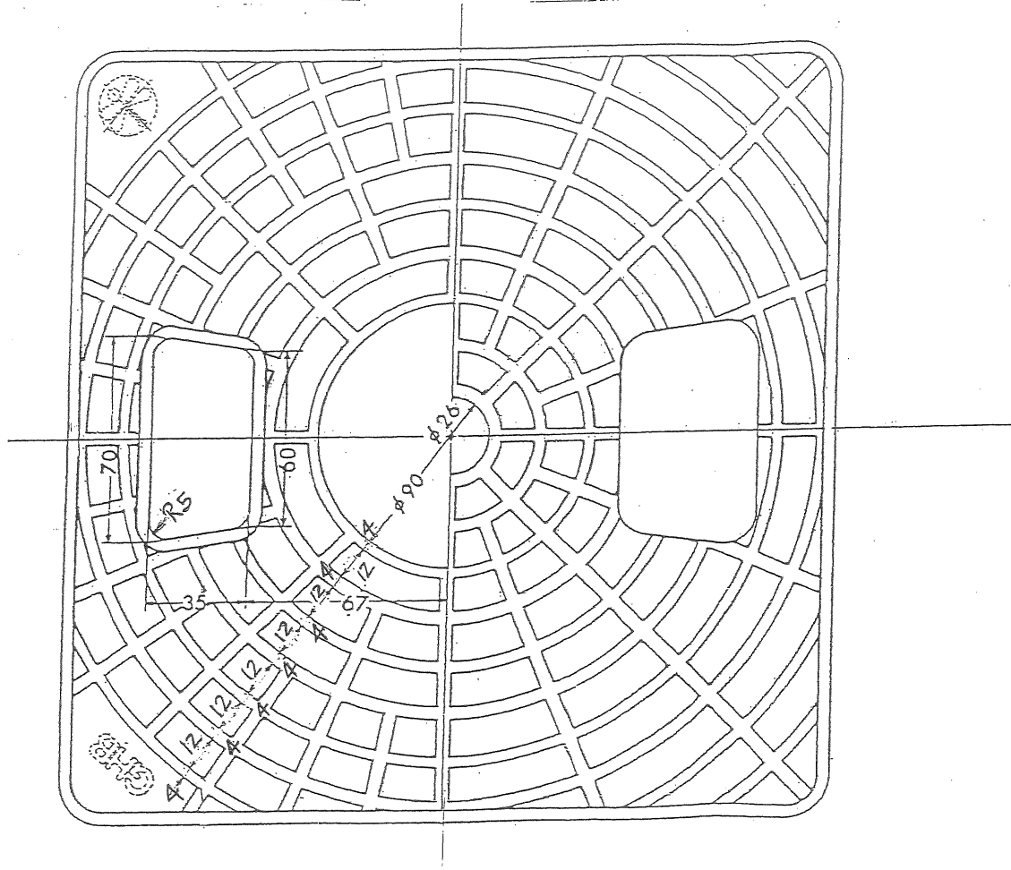
平面図
