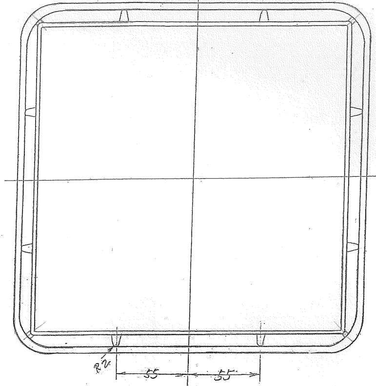
裏面図
