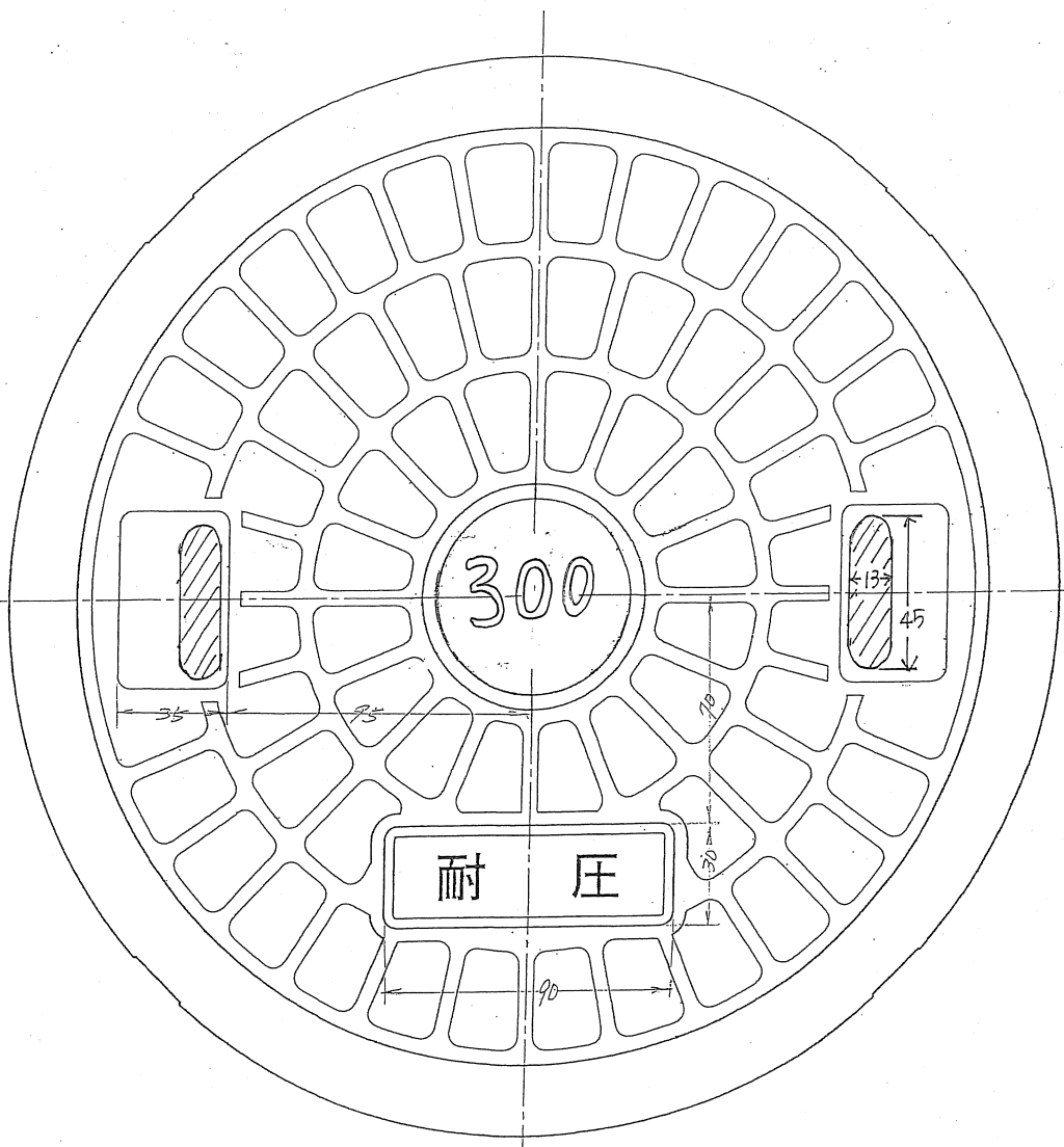
平面図
